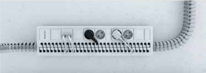
Duplo Kit blanco fijado a pared y vértebras acopladas. White Duplo Kit fixed to wall and connected vertebrae.
