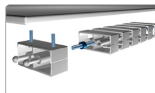
Easy-Steel bij starre montage
