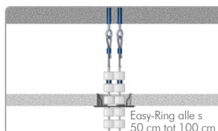
Plafondbevestiging Easy-Rope & Easy-Ring
