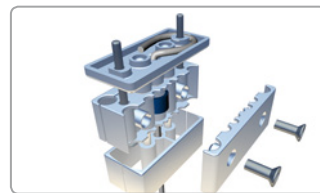
Klemfixering van de Easy-Rope
