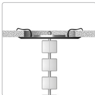
Bevestiging aan systeemplafond
