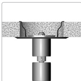
Krachtgeleiding systeemplafond tot 30 mm ik ben
