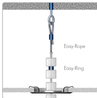
Bevestiging trekontlaster plafond
