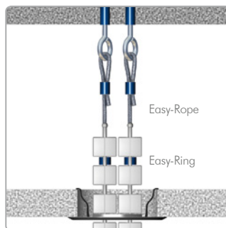
B 2x KS Cube aan bouwkundigplafond
