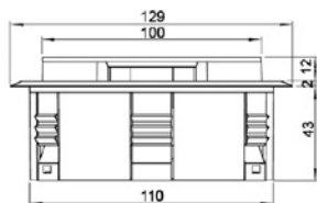
Easy-Outlet-TA voor geleiden een kabel
