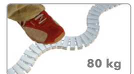
Belastbaarheid Gestrekt belastbaar: 80 kg, ineen-geschoven tot 100 kg
